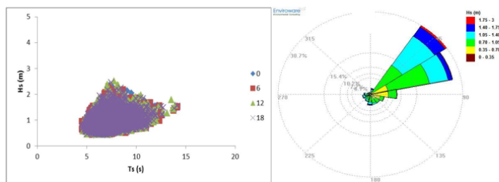
Gambar 4. Kondisi Gelombang di Pulau Marore; a. Karakteristik Gelombang; b. Mawar Gelombang
