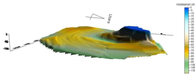
1 Gambar 7. Bentuk morfologi dasar laut di sekitar perairan Pulau Marore dari sisi Timur.
