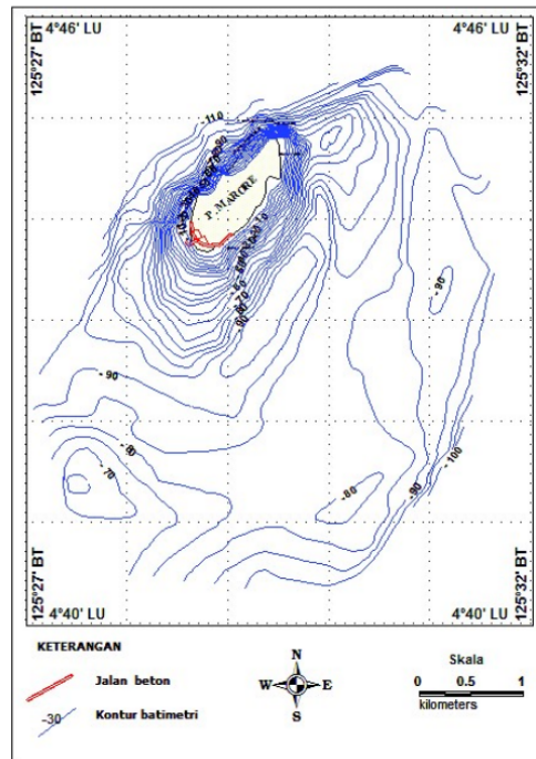
Gambar 6. Peta kontur kedalaman laut di perairan Pulau Marore. *Sumber: Rachmat & Purwanto, 2011.
