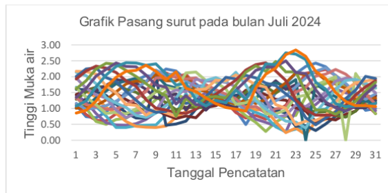
Gambar 5. Grafik pasang surut pada bulan Juli 2024.
