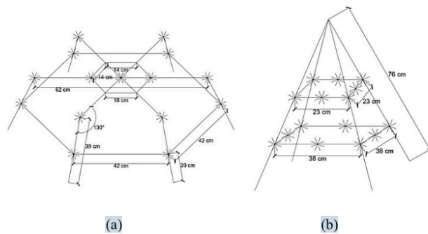
Gambar 1. Desain struktur transplantasi terumbu karang (a) model web spider dan (b) model pyramid
