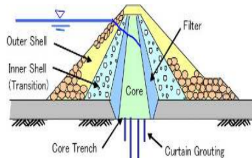
Gambar 2. Bendungan Tipe Urugan Centre Core Rock Fill Dam
