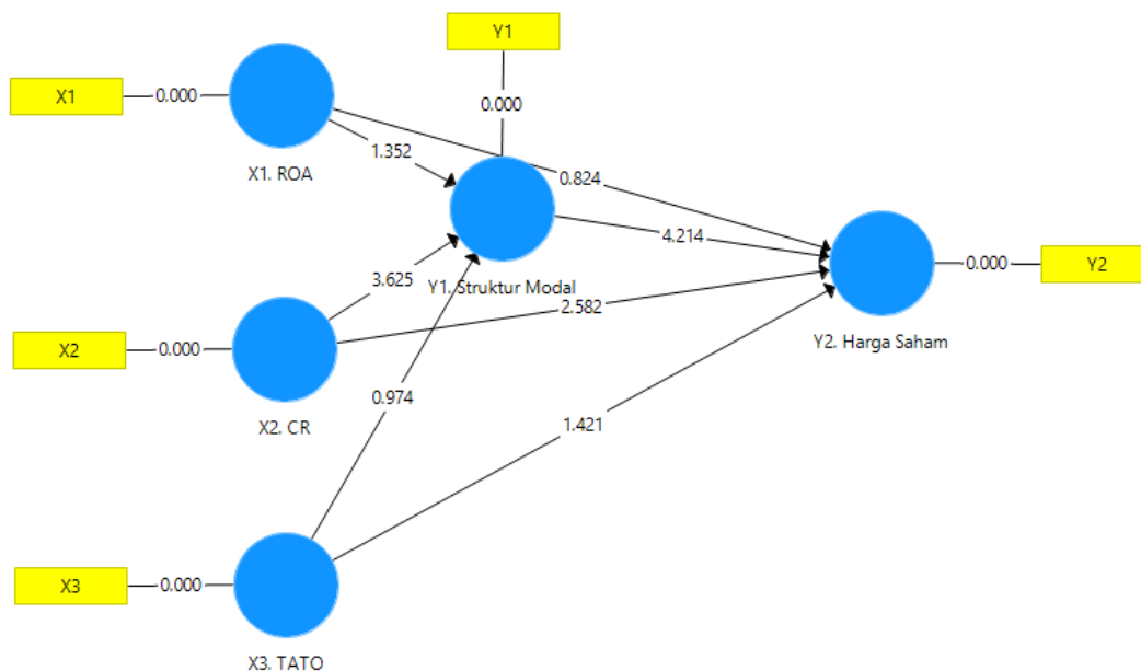
Gambar 2. Hasil Uji Model Struktural Melalui Aplikasi SmartPLS
