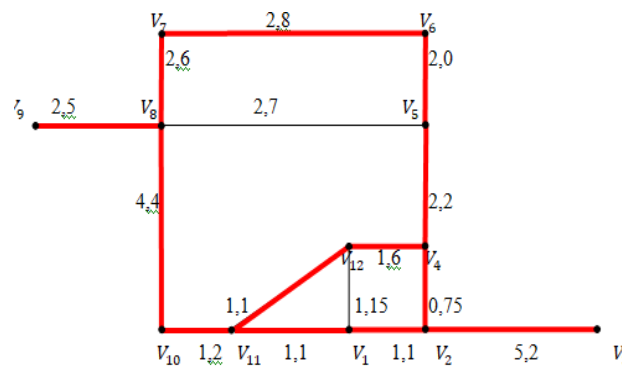
Gambar 15. Graf Rute Yang di Pilih Dari V_5 - V_3
